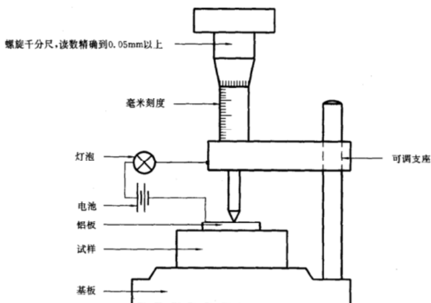
图 A1 测微计示意图
